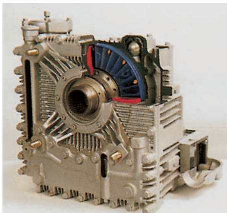
Σχ. 9.36 Υδραυλικός επιβραδυντής.
