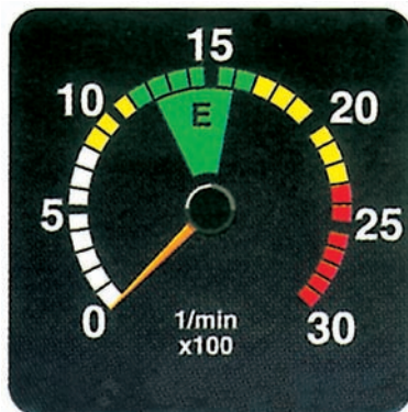
Σχ. 9.19 Στροφόμετρο.
