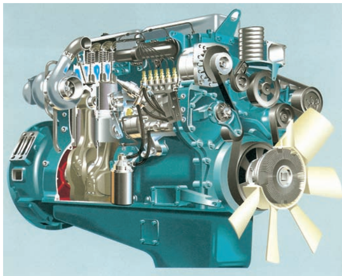
Σχ. 9.13 Πετρελαιοκινητήρας.
